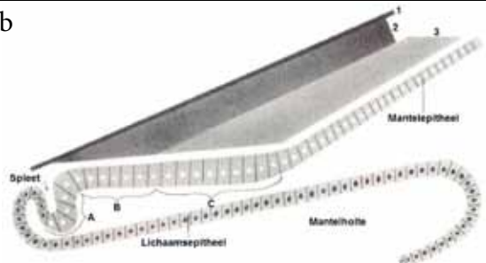
Afbeelding 4. Schelp en mantel. (a) Schematische verticale doorsnede van de schelp en mantel van een tweekleppige. (b) Vorming van de schelp. In zone A wordt het periostracum (1) afgescheiden. In zone B wordt de prismalaag (2) afgescheiden. In zone C wordt de porseleinlaag (3) afgescheiden.
